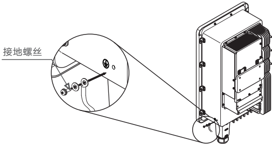
图5.9 线缆固定
