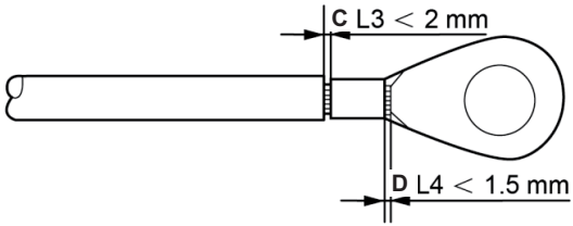
图5.8 线缆压接
