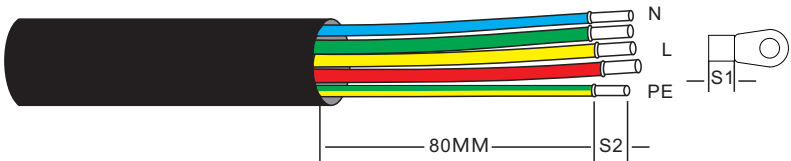
图 5.17 加工电缆线
