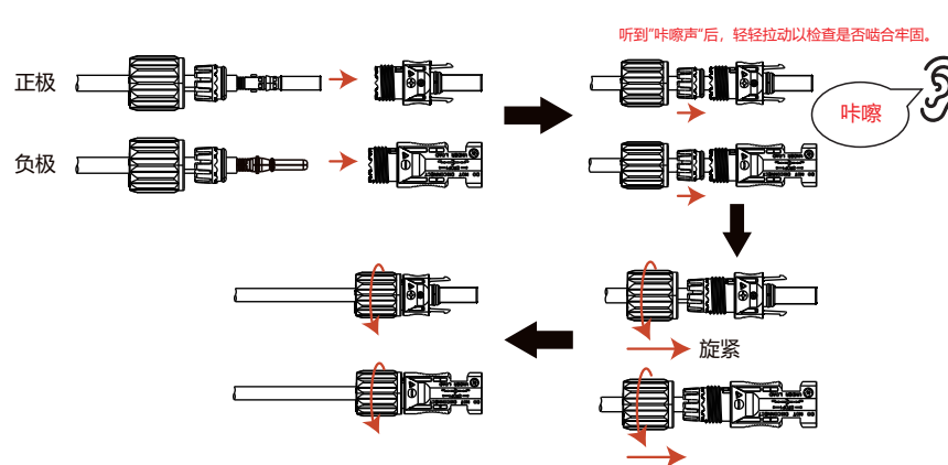
图5.14 组装连接器
