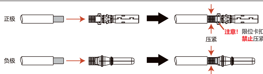
图5.13 压线
