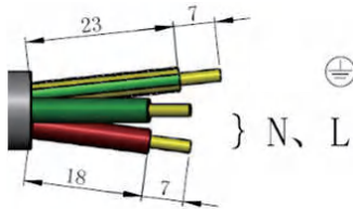
图4.14 交流线缆制作
