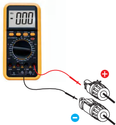
图4.12 万用表测量
