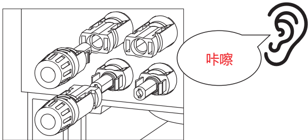
图4.13 连接到逆变器
