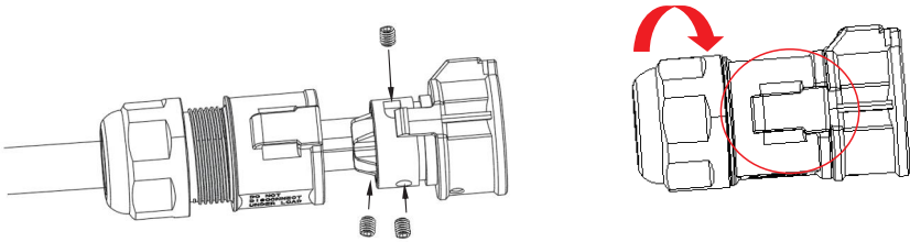
图4.22 连接电缆线
