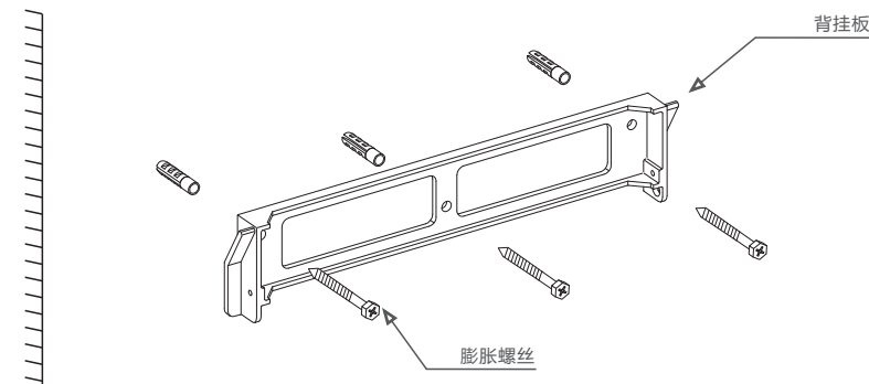
图4.4 逆变器安装
