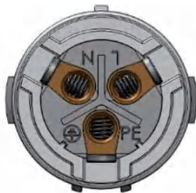
图4.16 交流端子内部示意图
