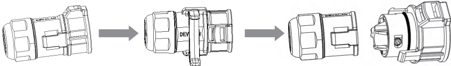
图4.21 拆开交流端子
