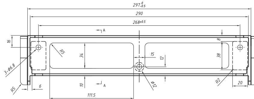
图4.3 背挂板尺寸
