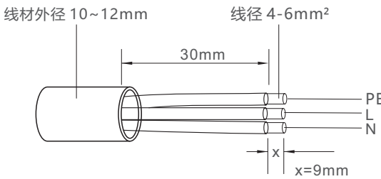
图4.20 剥线
