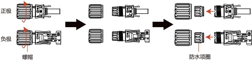
图4.7 拆卸连接器盖
