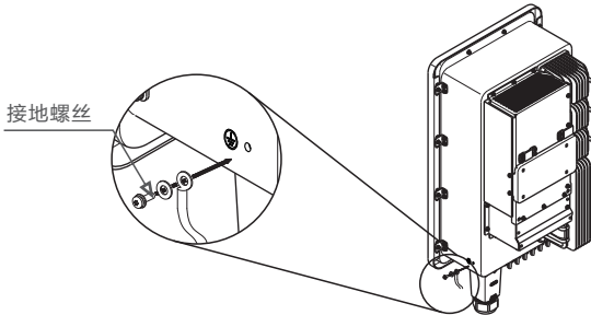
图5.9 线缆固定
