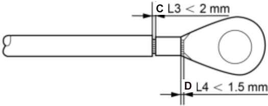
图5.9 线缆压接
