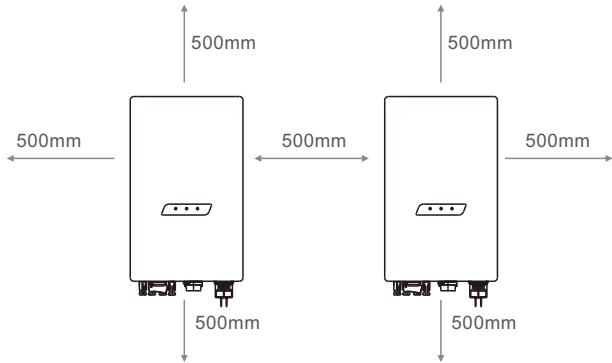
图5.2 逆变器的安装间隙
