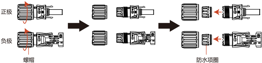
图5.12 拆卸连接器盖
