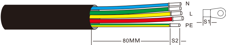
图 5.18 加工电缆线
