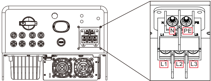
图5.19 逆变器交流端子
