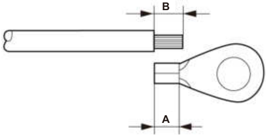
图5.8 剥线长度
